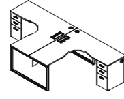
两人L工位主桌 DL62-2.CG W1400*D2812*H750 W1500*D3012*H750 W1600*D3212*H750
