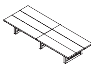
会议桌 EF78 Meeting Table W4800*D1800*H760 W3600*D1600*H760
