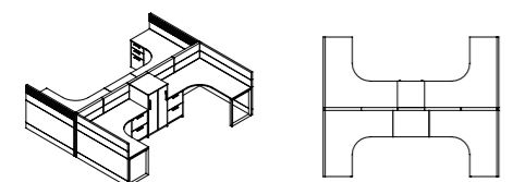
Vik66+vera42 工字型工作站 3884*3166*1150mm
