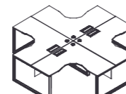
四人L工位主桌 DL63-2.GJ W2812*D2812*H750 W3012*D3012*H750 W3212*D3212*H750
