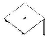
洽谈桌 DE720 1000(W)*1000(D)*750(H) 1200(W)*1200(D)*750(H) 1400(W)*1400(D)*750(H) 1500(W)*1500(D)*750(H) 1600(W)*1600(D)*750(H)
