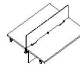
延伸工位 DE826 1200(W)*1226(D)*750(H) 1400(W)*1226(D)*750(H) 1500(W)*1426(D)*750(H) 1600(W)*1426(D)*750(H)
