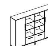
开门文件柜 DE87 2286(W)*427(D)*1584(H)
