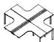
四人延伸工位 DE85FN-B 2826(W)*3020(D)*750(H) 3026(W)*3220(D)*750(H) 3226(W)*3420(D)*750(H)
