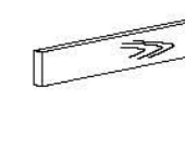
板式铝框屏 DELK 1200(W)*350(D)*28(H) 1300(W)*350(D)*28(H) 1400(W)*350(D)*28(H) 1500(W)*350(D)*28(H) 1600(W)*350(D)*28(H)
