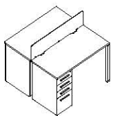
两人职员桌 DE82 1200(W)*1226(D)*750(H) 1400(W)*1426(D)*750(H) 1500(W)*1426(D)*750(H) 1600(W)*1626(D)*750(H)
