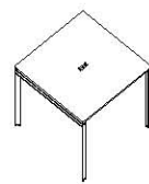
洽谈桌 DE70N 1000(W)*1000(D)*750(H) 1200(W)*1200(D)*750(H) 1400(W)*1400(D)*750(H) 1500(W)*1500(D)*750(H) 1600(W)*1600(D)*750(H)
