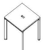
洽谈桌 DE71N 1000(W)*1000(D)*750(H) 1200(W)*1200(D)*750(H) 1400(W)*1400(D)*750(H) 1500(W)*1500(D)*750(H) 1600(W)*1600(D)*750(H)
