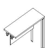
延伸桌 DE825H 1200(W)*400(D)*750(H) 1400(W)*400(D)*750(H)
