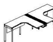
两人延伸工位 DE82FN-B 1400(W)*3020(D)*750(H) 1500(W)*3220(D)*750(H) 1600(W)*3420(D)*750(H)
