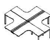
四人延伸工位 DE85FN-A 2826(W)*3020(D)*750(H) 3026(W)*3220(D)*750(H) 3226(W)*3420(D)*750(H)
