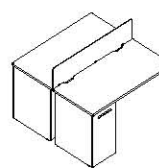
两人职员桌 DE83 1200(W)*1226(D)*750(H) 1400(W)*1426(D)*750(H) 1500(W)*1426(D)*750(H) 1600(W)*1626(D)*750(H)
