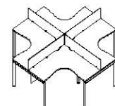
四人工位 DE85 2826(W)*2826(D)*750(H) 3026(W)*3026(D)*750(H) 3226(W)*3226(D)*750(H)
