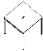
洽谈桌 DE70N 1000(W)*1000(D)*750(H) 1200(W)*1200(D)*750(H) 1400(W)*1400(D)*750(H) 1500(W)*1500(D)*750(H) 1600(W)*1600(D)*750(H)
