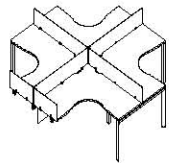
延伸工位 DE825 2852(W)*2826(D)*750(H) 3052(W)*3026(D)*750(H) 3252(W)*3226(D)*750(H)
