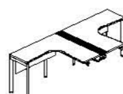
两人延伸工位 DE82FN-B 1400(W)*3020(D)*750(H) 1500(W)*3220(D)*750(H) 1600(W)*3420(D)*750(H)
