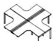
四人延伸工位 DE85FN-B 2826(W)*3020(D)*750(H) 3026(W)*3220(D)*750(H) 3226(W)*3420(D)*750(H)
