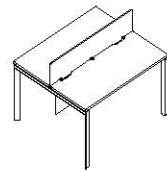
两人工位 DE86 1200(W)*1226(D)*750(H) 1400(W)*1226(D)*750(H) 1500(W)*1426(D)*750(H) 1600(W)*1426(D)*750(H)
