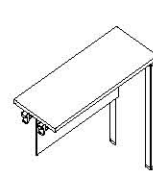
延伸桌 DE825H 1200(W)*400(D)*750(H) 1400(W)*400(D)*750(H)
