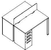
两人职员桌 DE82 1200(W)*1226(D)*750(H) 1400(W)*1426(D)*750(H) 1500(W)*1426(D)*750(H) 1600(W)*1626(D)*750(H)
