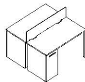
两人职员桌 DE83 1200(W)*1226(D)*750(H) 1400(W)*1426(D)*750(H) 1500(W)*1426(D)*750(H) 1600(W)*1626(D)*750(H)
