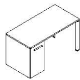
职员桌 DE81 1200(W)*800(D)*750(H) 1400(W)*700(D)*750(H) 1500(W)*700(D)*750(H) 1600(W)*800(D)*750(H)
