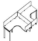
延伸工位 DE822 1452(W)*2826(D)*750(H) 1552(W)*3026(D)*750(H) 1652(W)*3226(D)*750(H)
